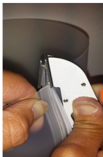
5. Insérer la glissière gauche sur la partie oblique au fond de la gorge gauche de l'outil, comme pour une fermeture éclair classique.
